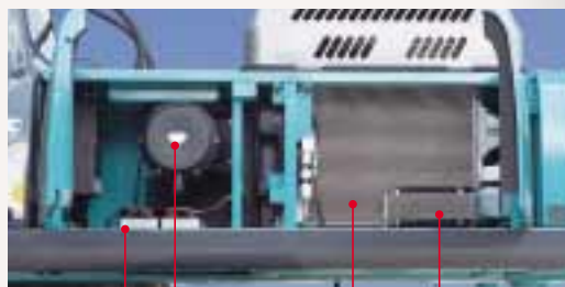
バッテリー エアクリーナ インタークーラ 燃料クーラ
