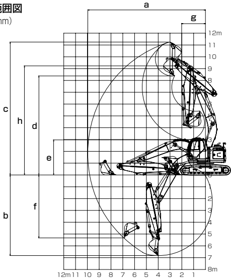
■作動範囲図 左 SK225SR/右 SK235SR (単位: mm)
