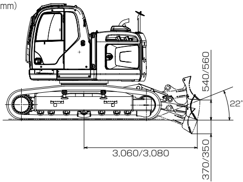
■作動範囲図 左 SK225SR/右 SK235SR (単位: mm)
