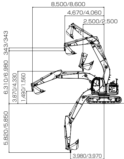
■作動範囲図 左 SK225SR/右 SK235SR[LC] (単位: mm)
